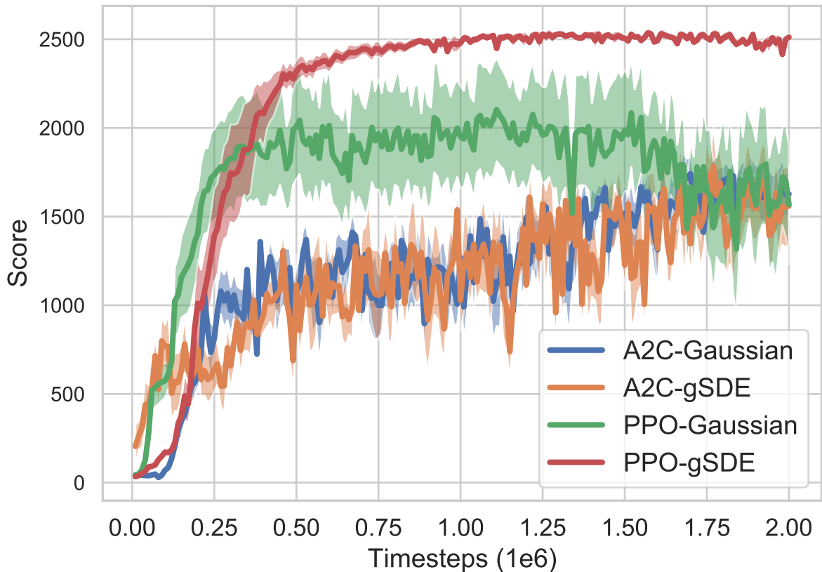
HopperBulletEnv-v0
