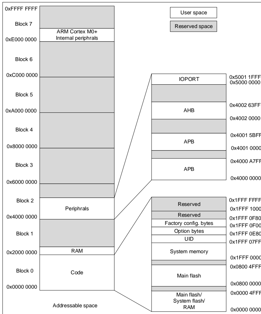
图 3-2 存储器映射
