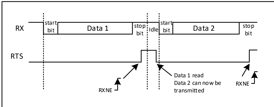
图 20-14 RTS 流控制
