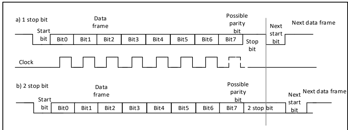
图 20-3 配置停止位
