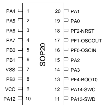
图 3-8 SOP20 Pinout1 PY32F003F1xS
