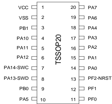
图 3-7 TSSOP20 Pinout6 PY32F003F6xP
