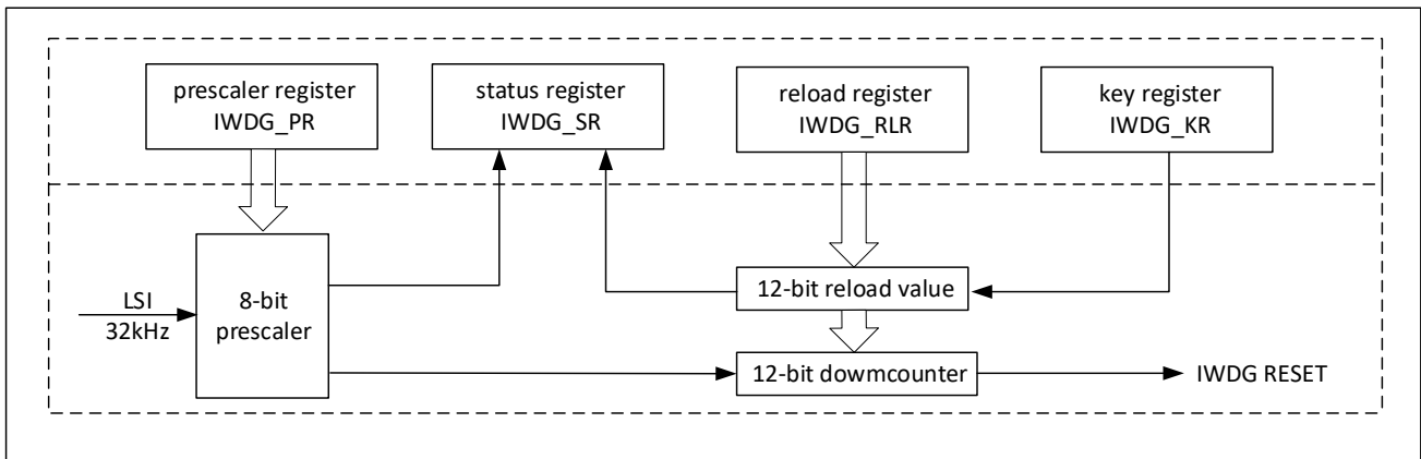
图 22-1 IWDG 框图
