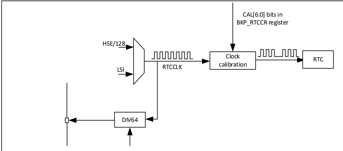
图 24-4 RTC 校准图
