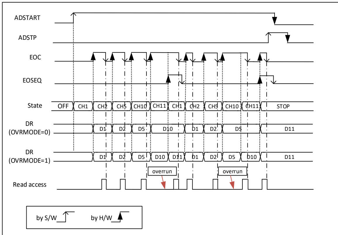
图 14-10 过载
