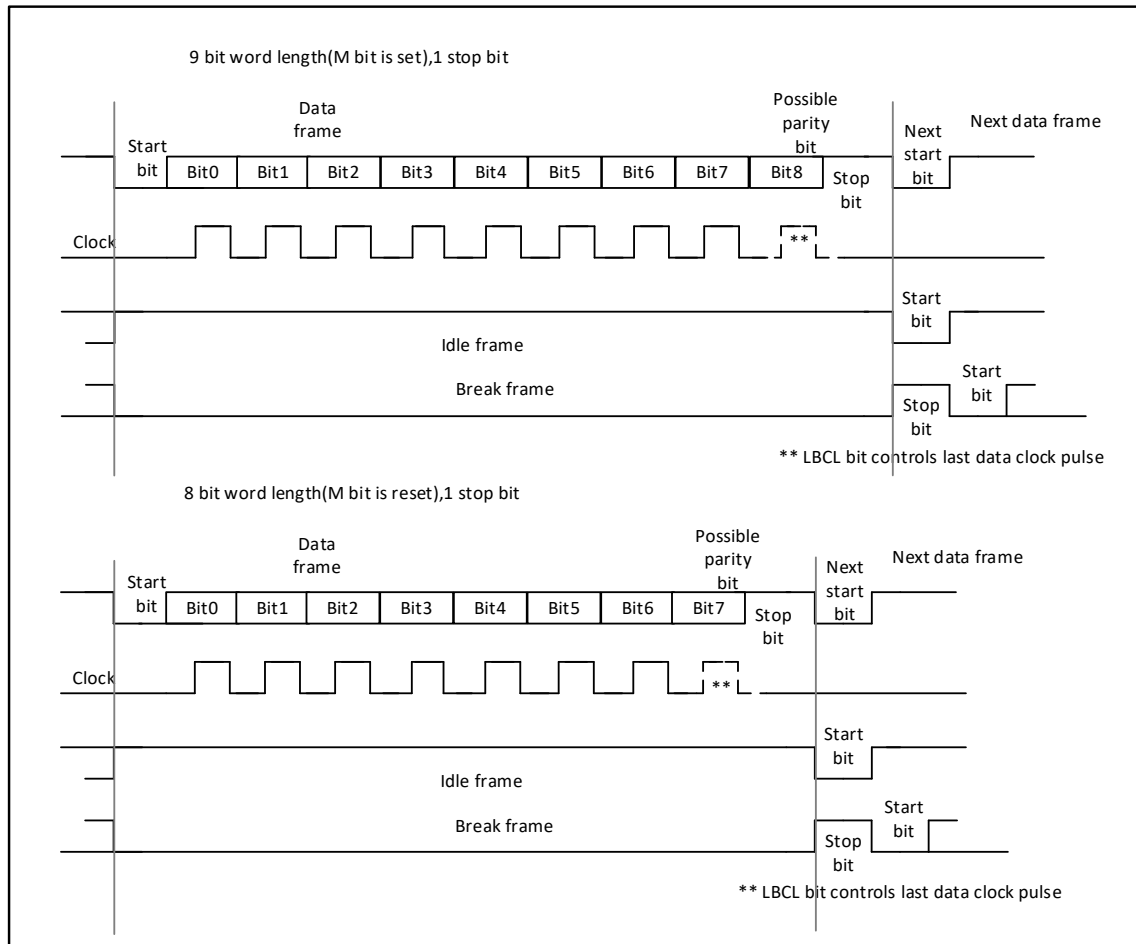
图 26-2 字长设置
