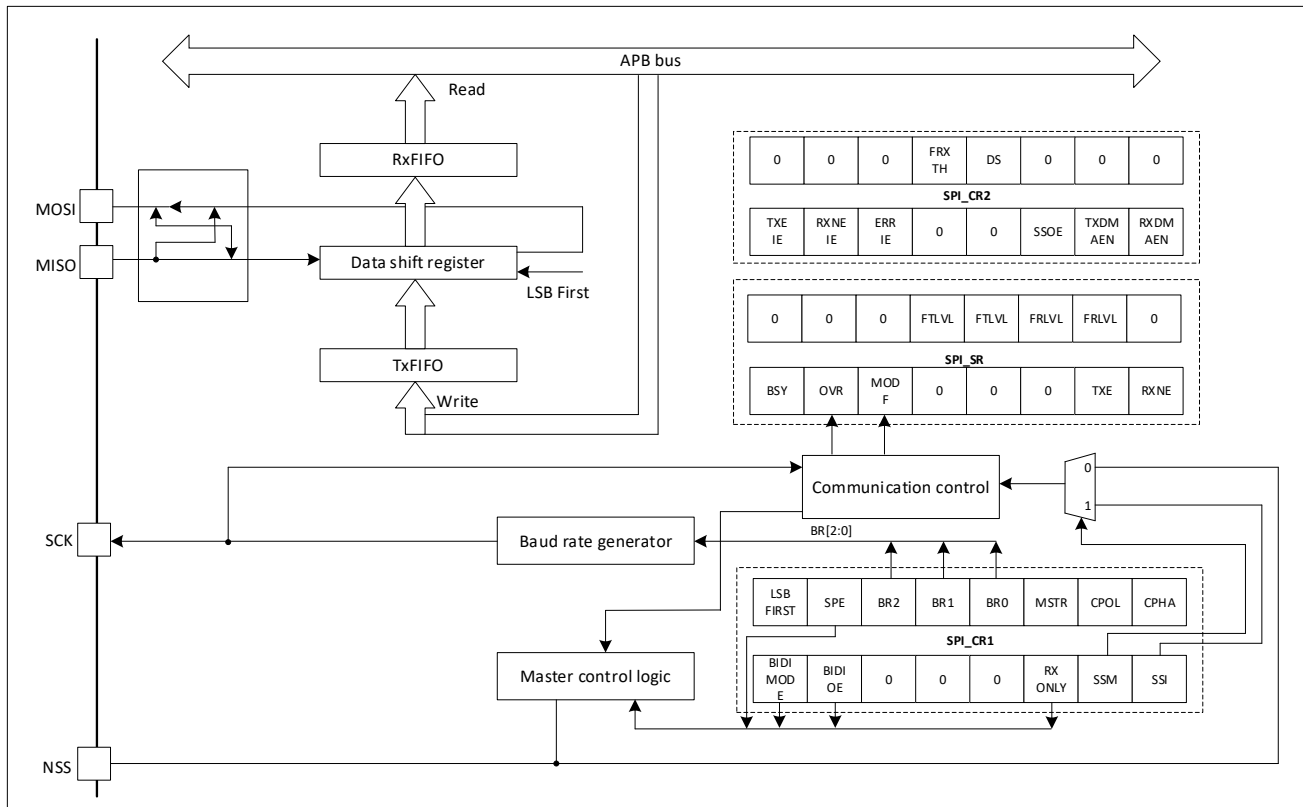
图 27-1 SPI 框图
