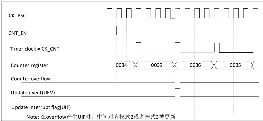
图 16-17 计数器时序图, 内部时钟分频因子为 4, TIMx_ARR=0x36
