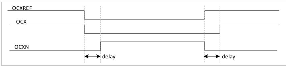
图 19-17 带死区插入的互补输出
