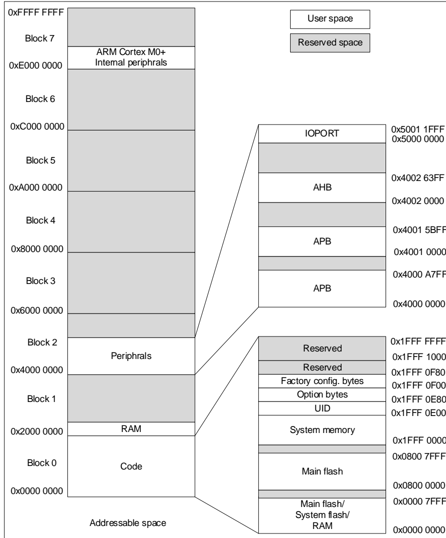
图 3-2 存储器映射
