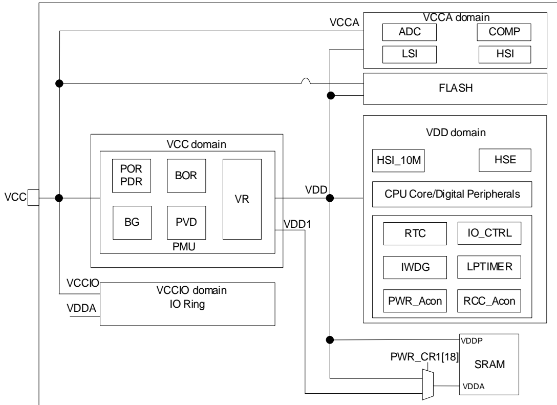
图 5-1 电源框图
