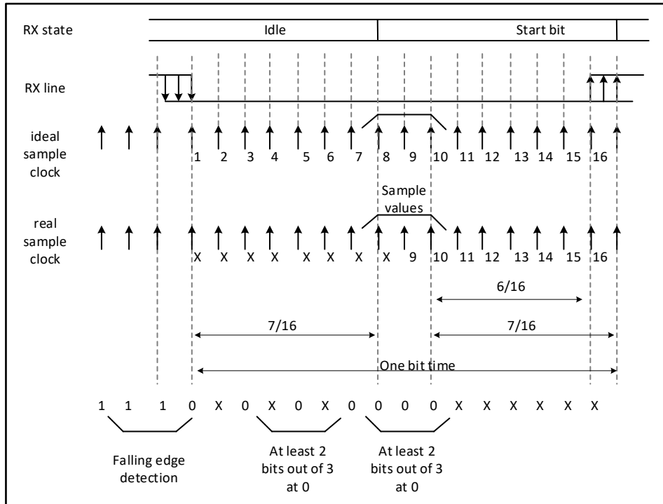
图 26-5 起始位检测
