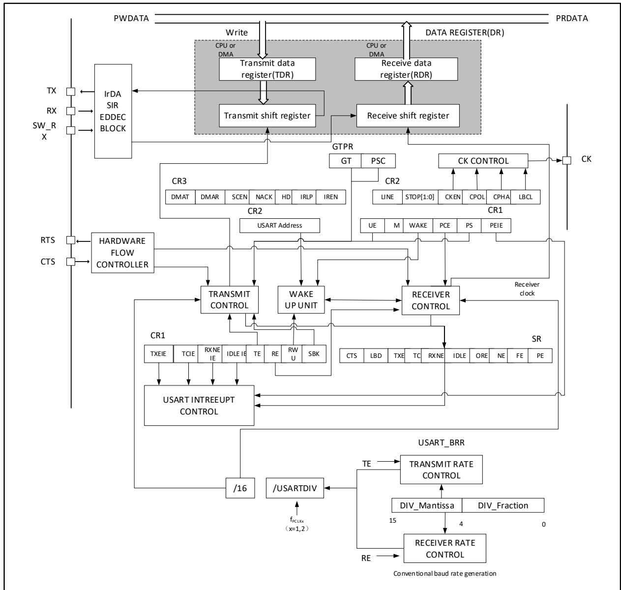
图 26-1 USART 框图
