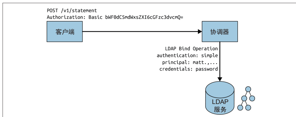
图 10-2: 使用外部 LDAP 服务对 Presto 进行 LDAP 认证
