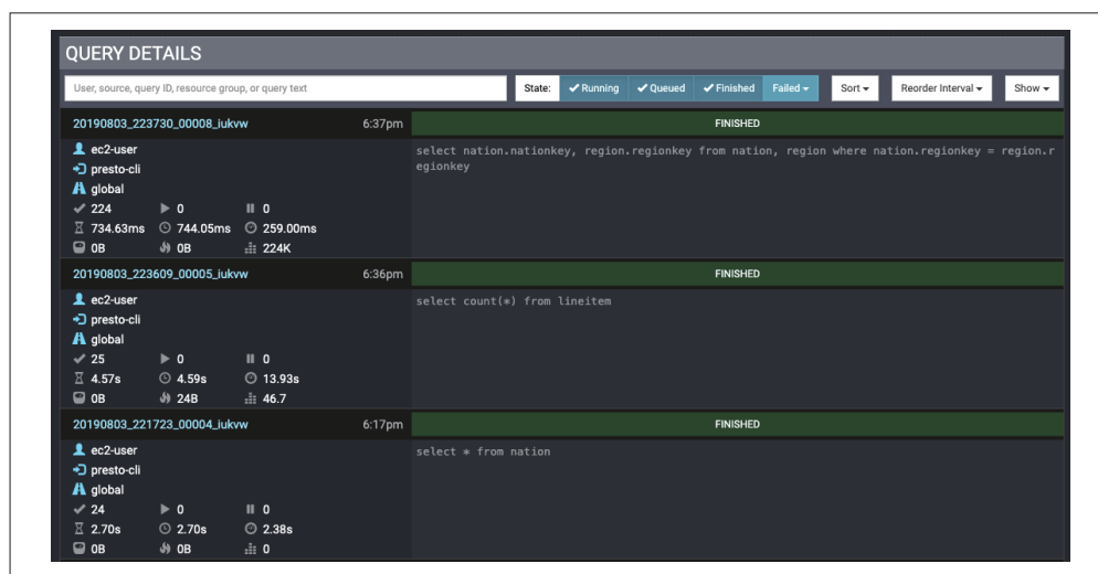
图 12-2: Presto Web UI 中的查询列表
