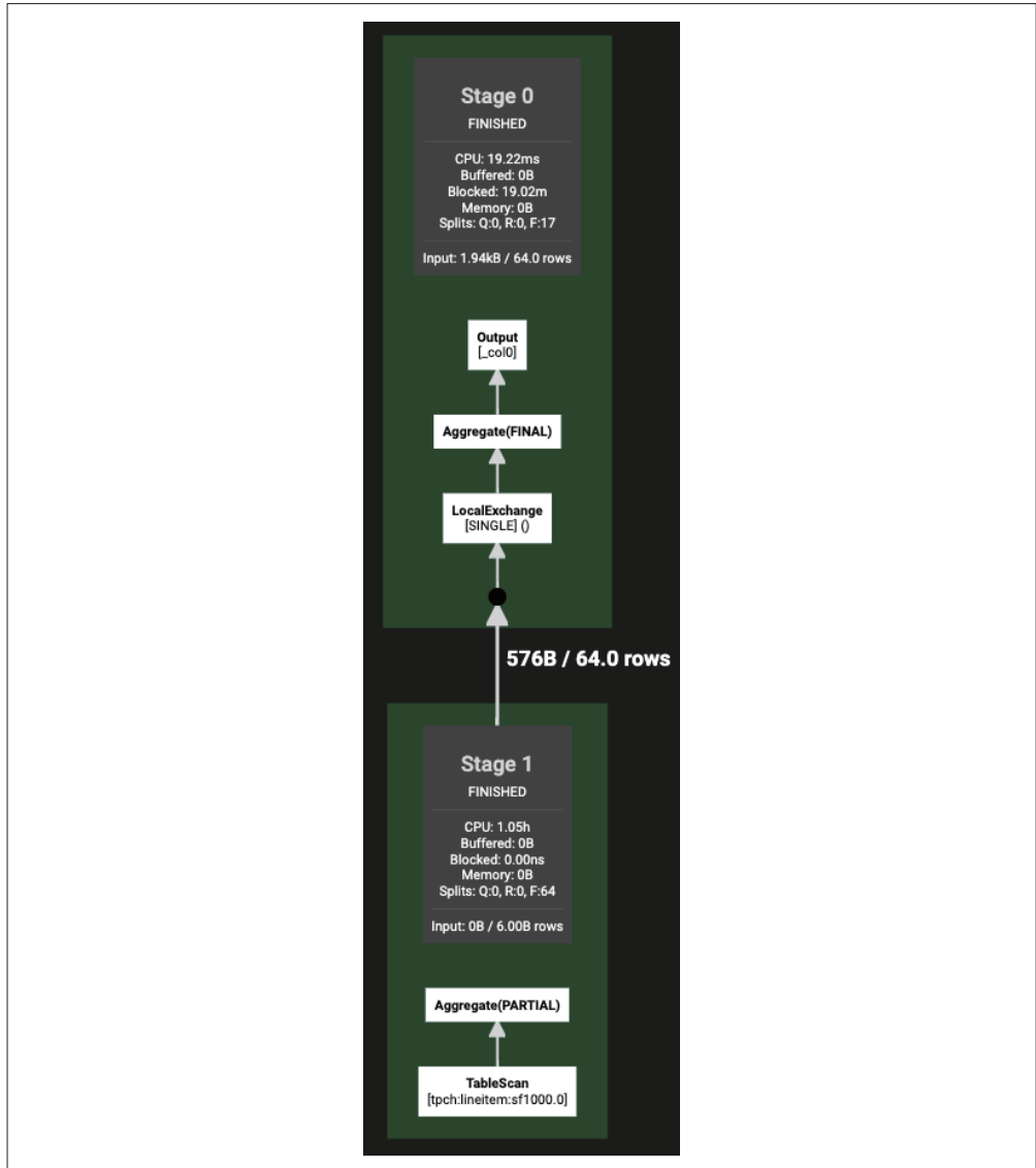
图 12-7：在 lineitem 上执行 count(*) 查询的实时计划示例
