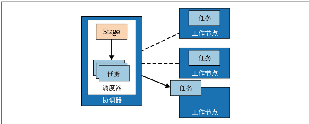
图 4-9: 协调器执行的任務管理
