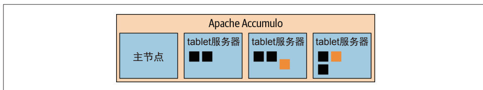
图 7-3: 具有主节点和多个 tablet 服务器的 Accumulo 架构
