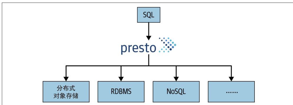
图 1-3: Presto 对多种数据源的 SQL 支持
