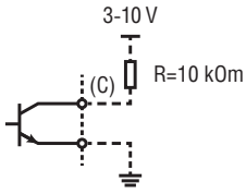
Схема подключения импульсного кабеля
