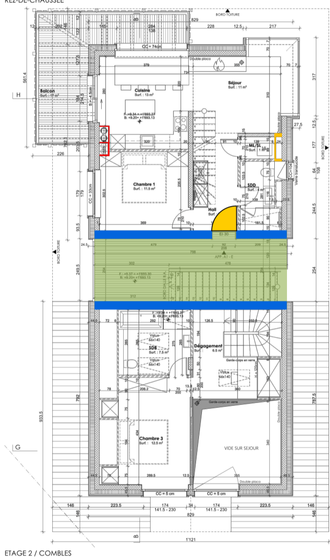
ETAGE 2 / COMBLES
