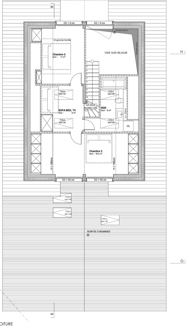
COMBLES / TOITURE
