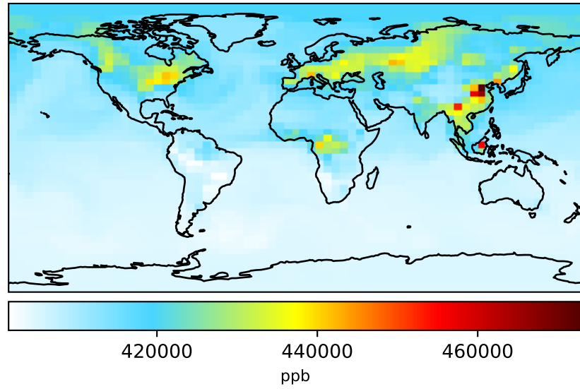
carbon_co2 (Dev) 4.0x5.0
