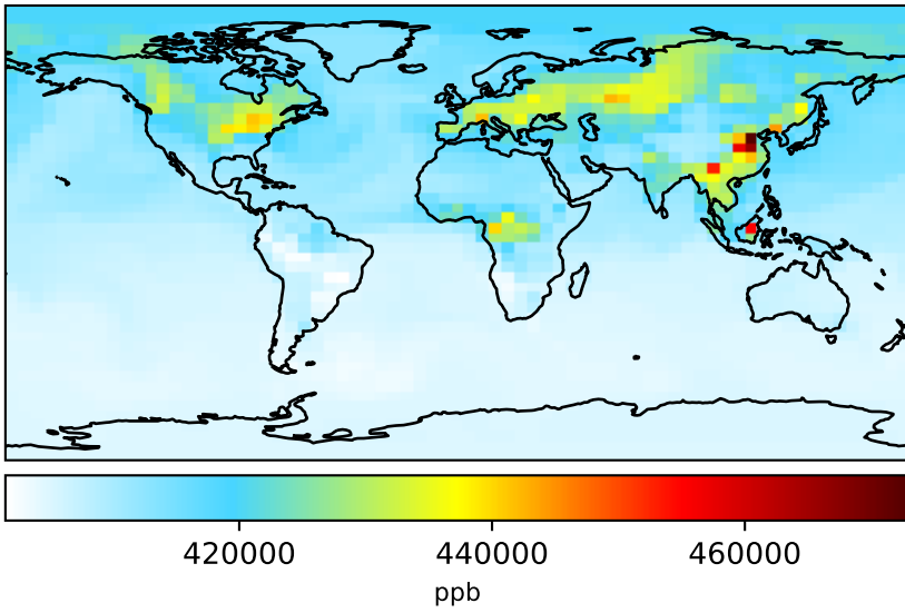
gcc_carbon (Ref) 4.0x5.0
