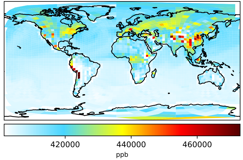
gchp_carbon (Dev) c24
