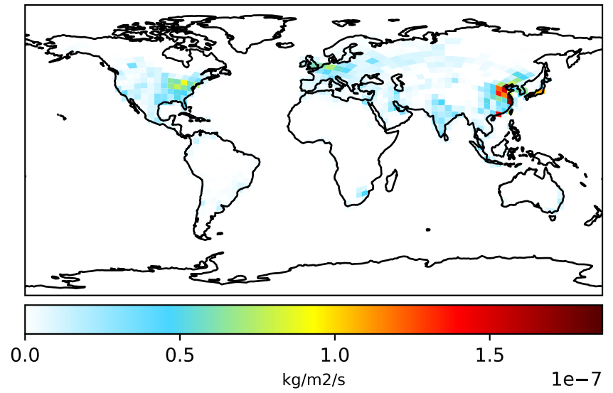
gchp_carbon-CO2 (Dev) c24
